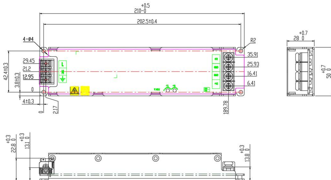
输入、输出端子定义及安装注意事项
